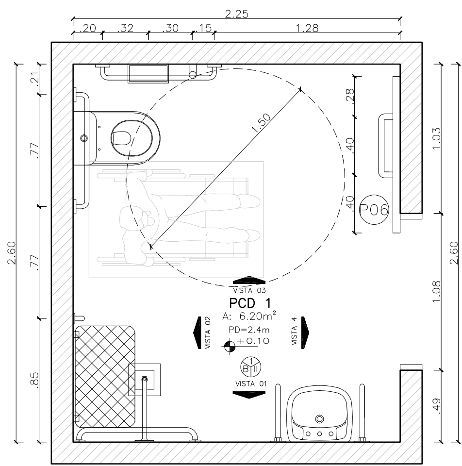
PLANTA BAIXA - SANITÁRIO PNE 1
