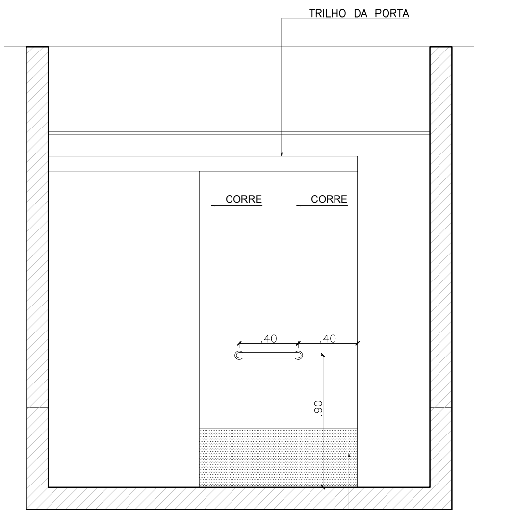
VISTA 04 - SANITÁRIO PNE 1
