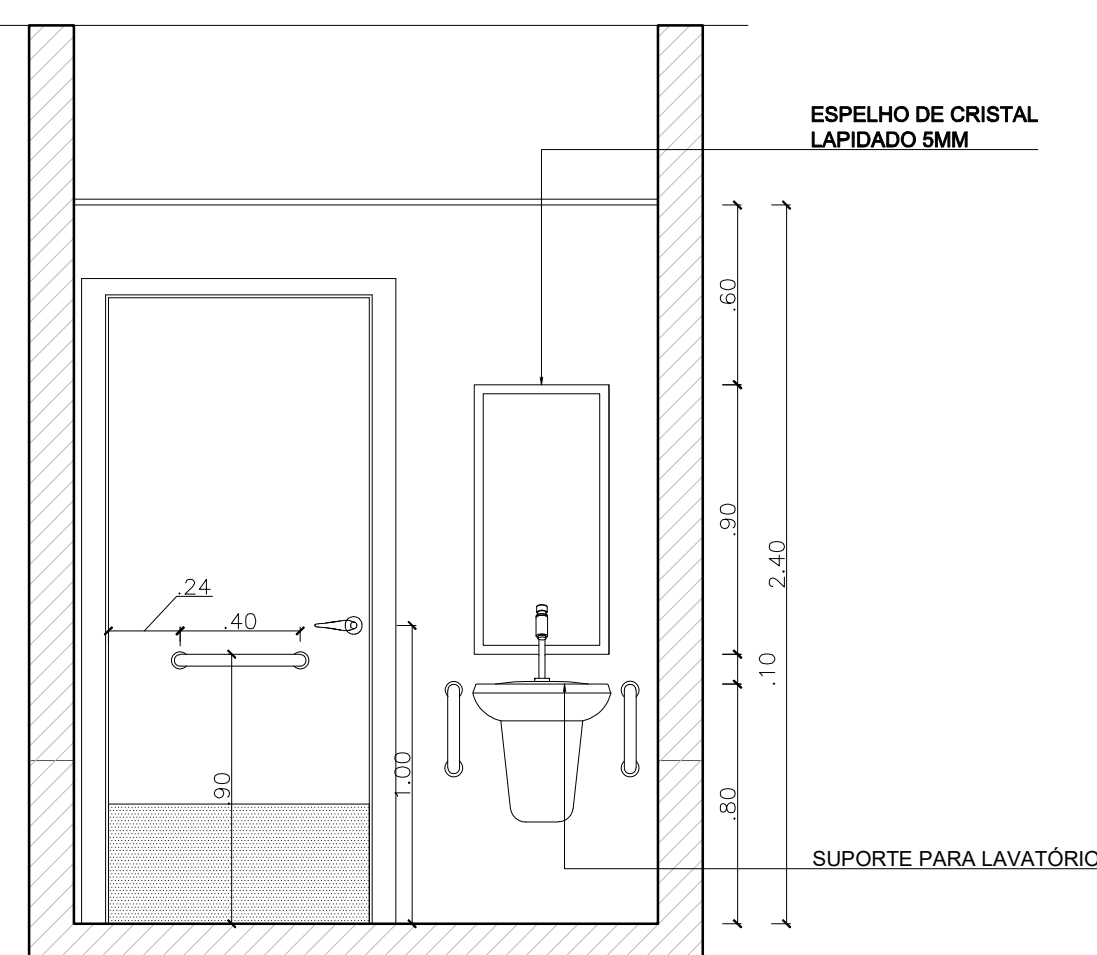
VISTA 03 - SANITÁRIO PNE 2
