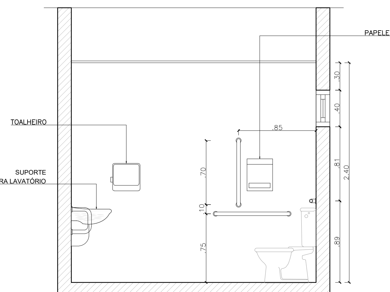
VISTA 04 - SANITÁRIO PNE 2
