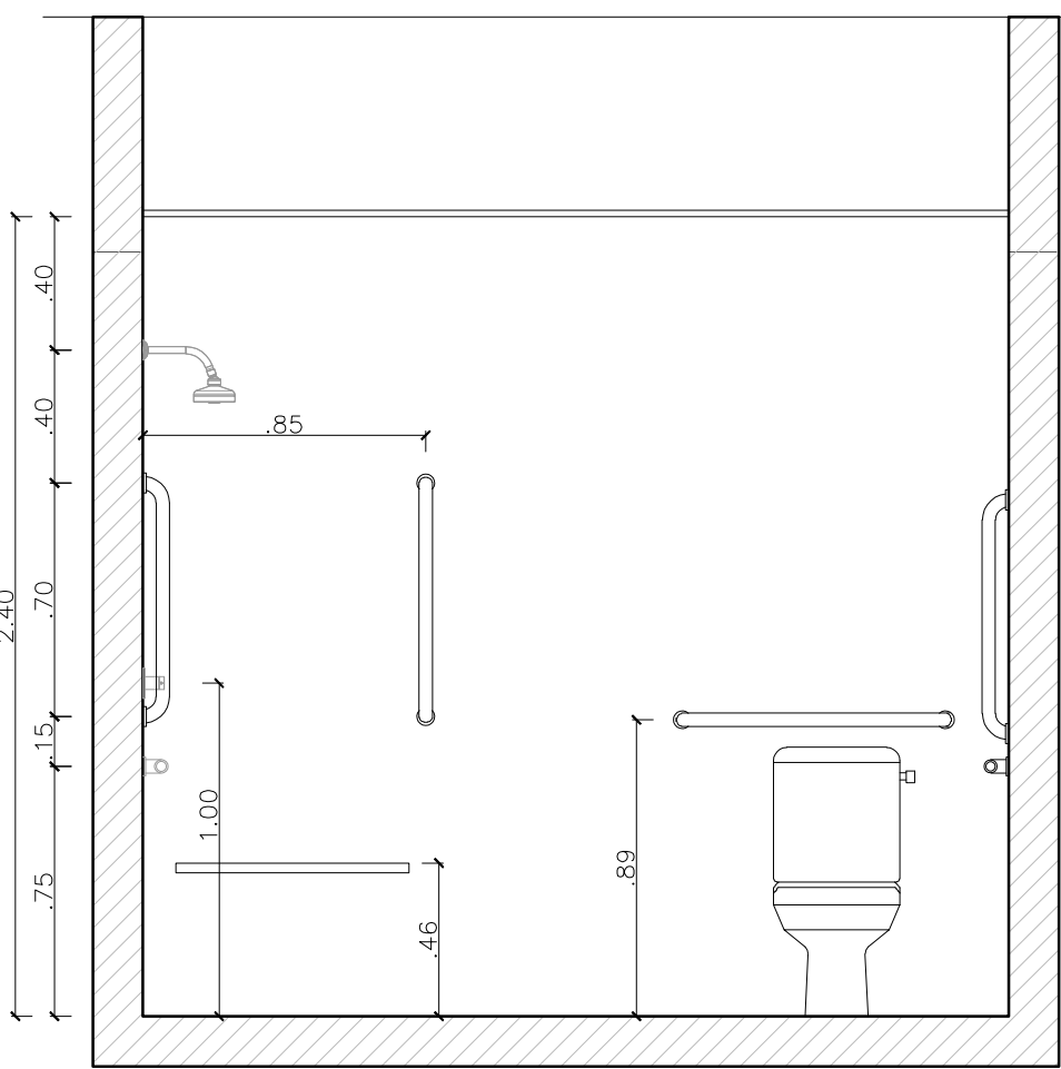
VISTA 02 - SANITÁRIO PNE 1
