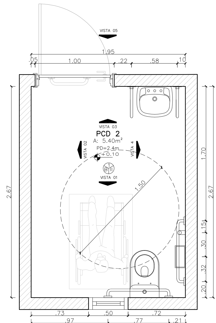
PLANTA BAIXA - SANITÁRIO PNE 2
