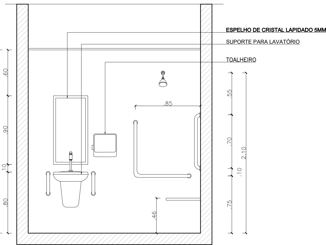
VISTA 01 - SANITÁRIO PNE 1
