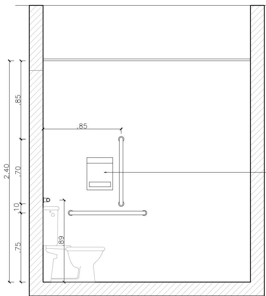
VISTA 03 - SANITÁRIO PNE 1
