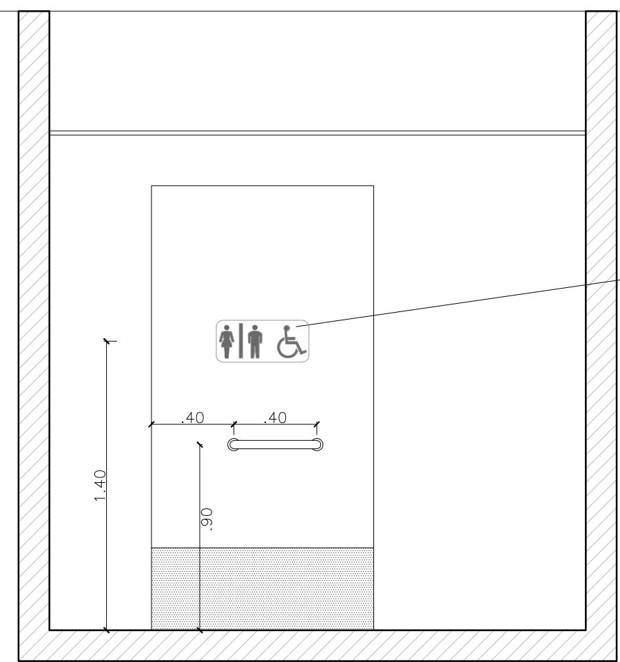
VISTA 05 - SANITÁRIO PNE 1
