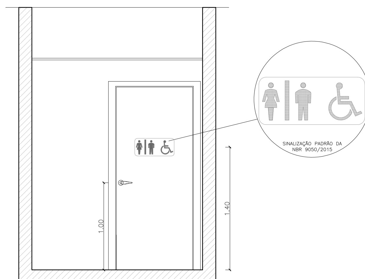
VISTA 05 - SANITÁRIO PNE 2
