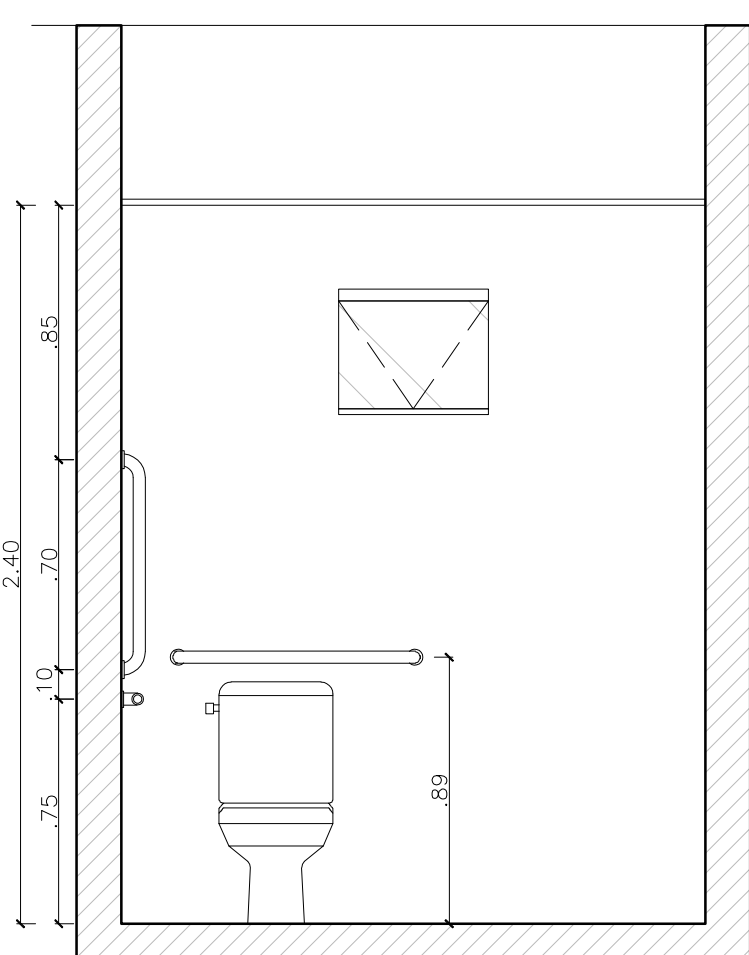
VISTA 01 - SANITÁRIO PNE 2
